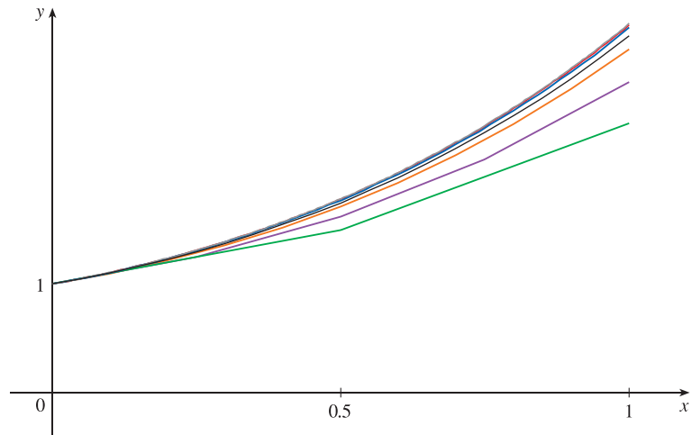
그림 15 정확한 해에 접근하는 오일러 근사식들
