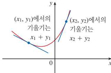
그림 1 y' = x + y 의 해
