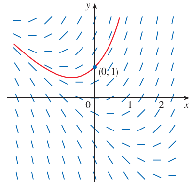
그림 4 (0, 1) 을 지나는 해곡선
